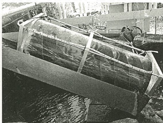
(マイクロ水力発電装置の実証実験現場)
