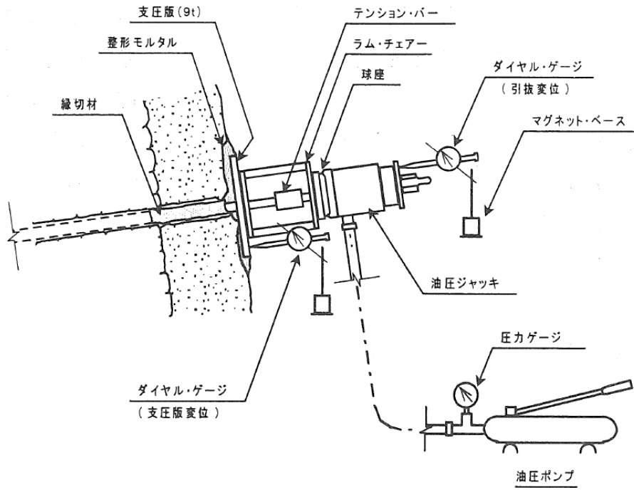
図一 2 試験概要図
