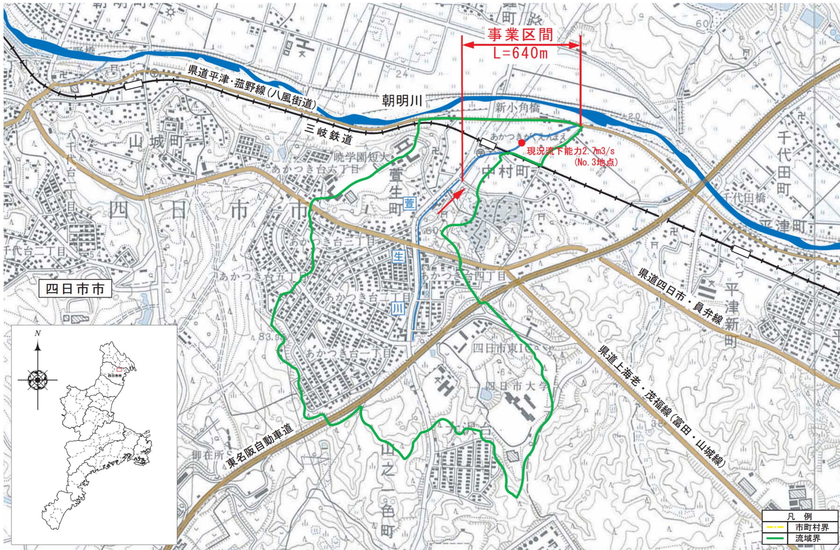
萱生川流域図、位置図 S=1:10,000
