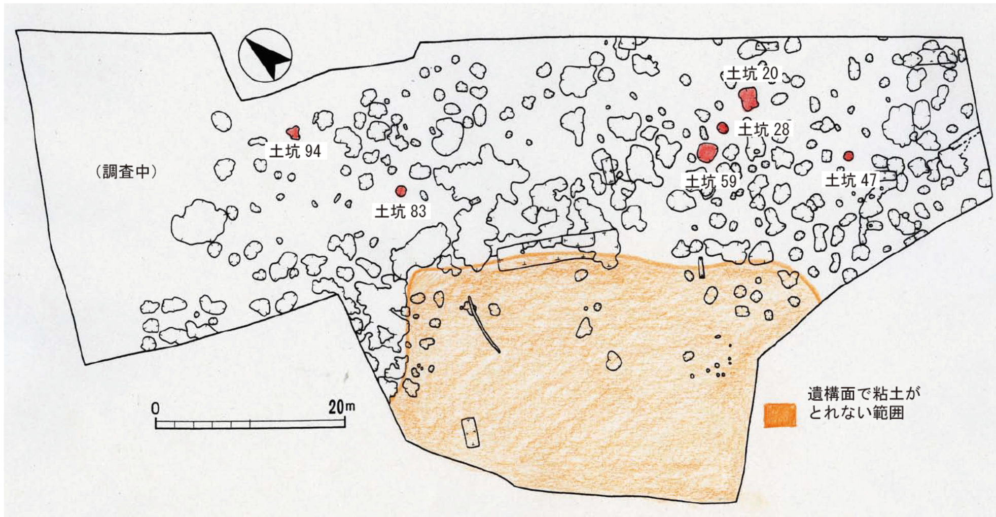
遺構平面図 1:400
