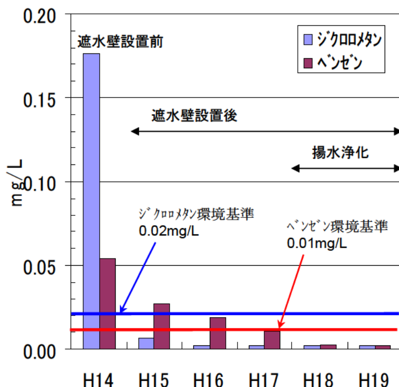
図 2.3 遮水壁外における全井戸のジクロロメタンとベンゼンの年平均濃度
