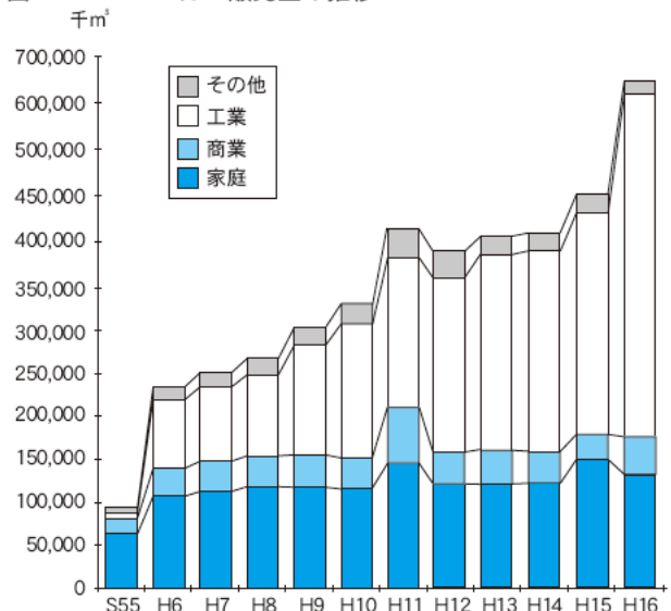
図1 2 3 ガス販売量の推移
