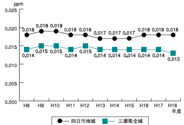
図1-3-2 二酸化窒素の経年変化
