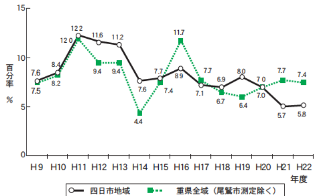
図1-3-4 光化学オキシダント昼間値(5~20時)が 0.06\text{ppm} を超えた時間数の割合の経年変化
