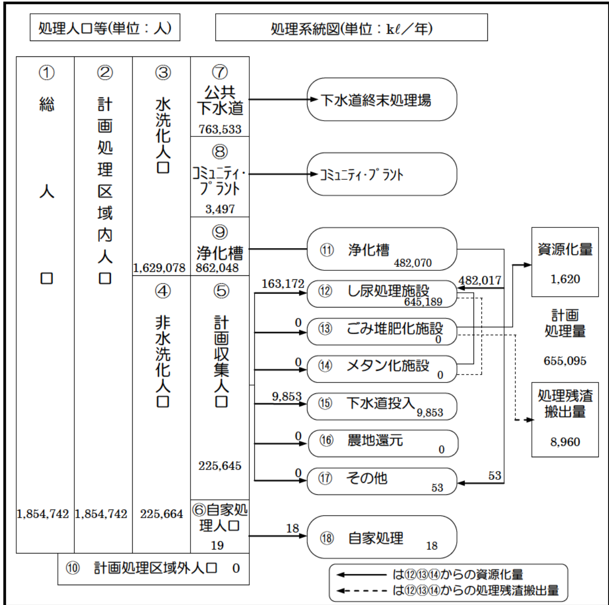
資料7-11 し尿処理のフロー図（平成22年度）
