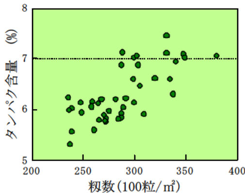
図1 「みえのえみ」の籾数とタンパクの関係 (H10, 11)
