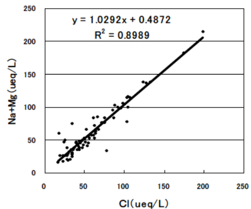
図 12 \text{Na}+\text{Mg}/\text{Cl} (n=76)
