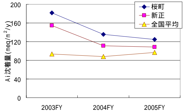
図 9 Ai 沈着量の推移
