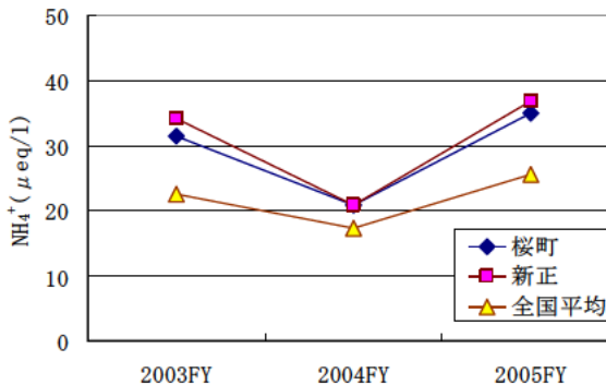
図6 \text{NH}_4^+ 濃度の年度平均比較
