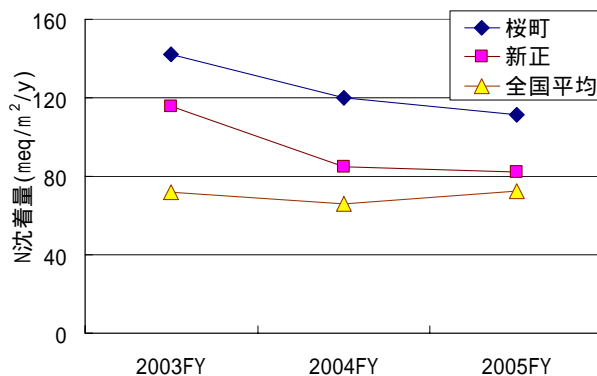
図 10 N 沈着量の推移
