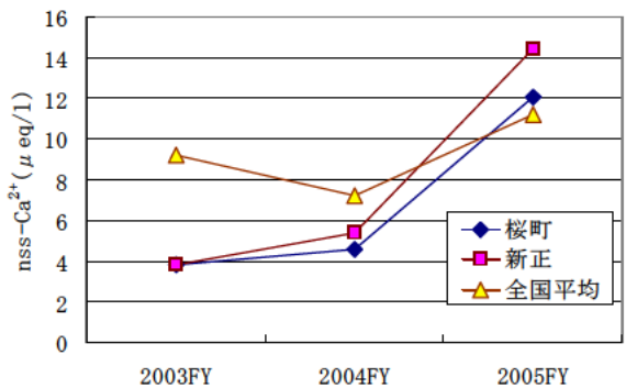
図7 \text{nss-Ca}^{2+} 濃度の年度平均比較
