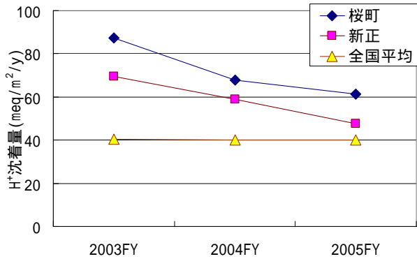
図 8 H + 沈着量の推移
