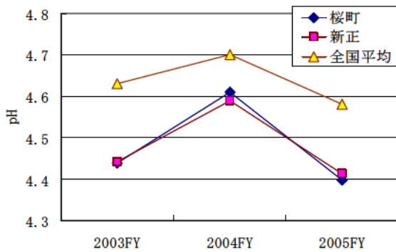
図2 pHの年度平均比較
