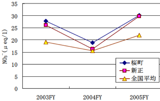
図4 \text{NO}_3^- 濃度の年度平均比較
