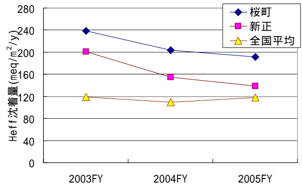
図 11 Heff 沈着量の推移
