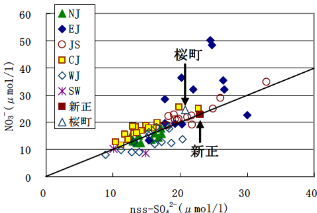
図 1 5 nss- \text{SO}_4^{2-} 濃度と \text{NO}_3^- 濃度の関係
