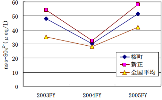
図5 \text{nss-SO}_4^{2-} 濃度の年度平均比較
