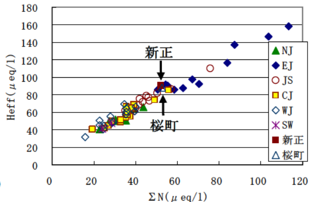
図 1 6 \Sigma\text{N} 濃度と \text{Heff} 濃度の関係
