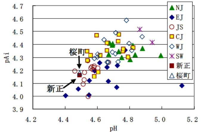
図 1 4 pH と pAi の関係
