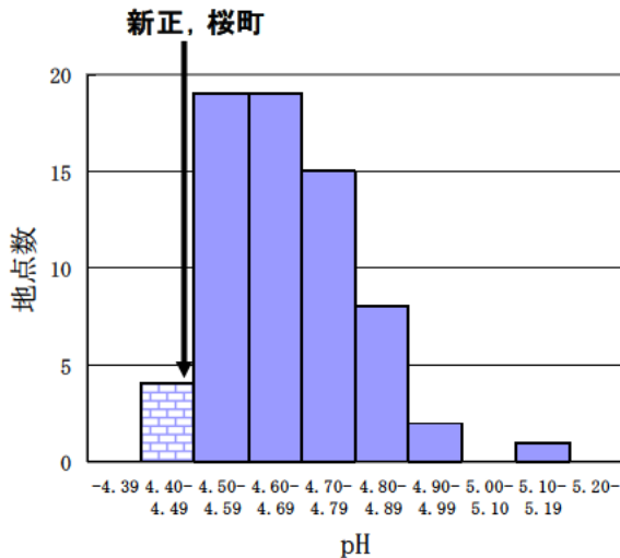
図 1 3 全国 pH の分布
