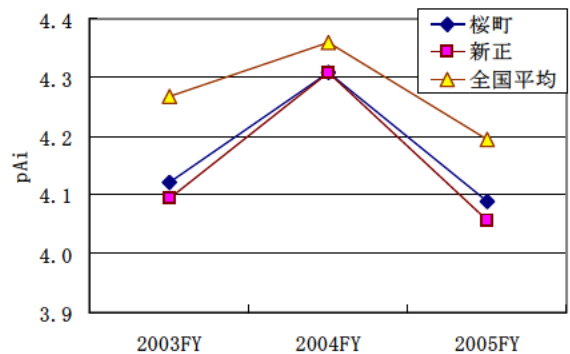
図3 pAiの年度平均比較
