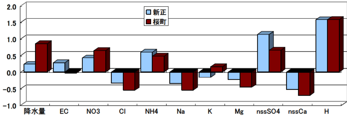
図 1 2 Zスコア(降水量及び各成分濃度)
