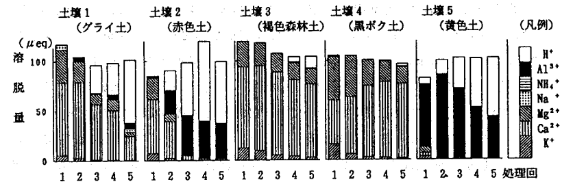
図2 pH3人工酸性雨流下 100ml毎の陽イオン溶脱量
