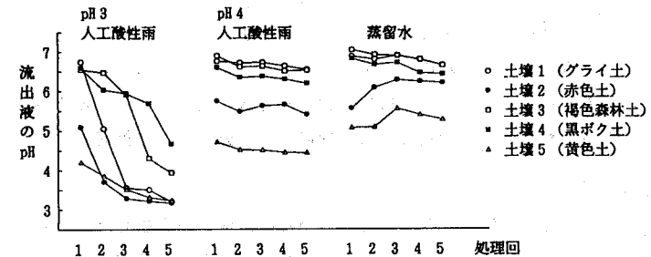
図1 土壌カラム流出液のpHに対する人工酸性雨処理の影響
