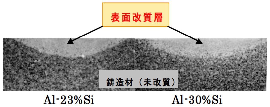
レーザー照射した断面のマクロ組織
