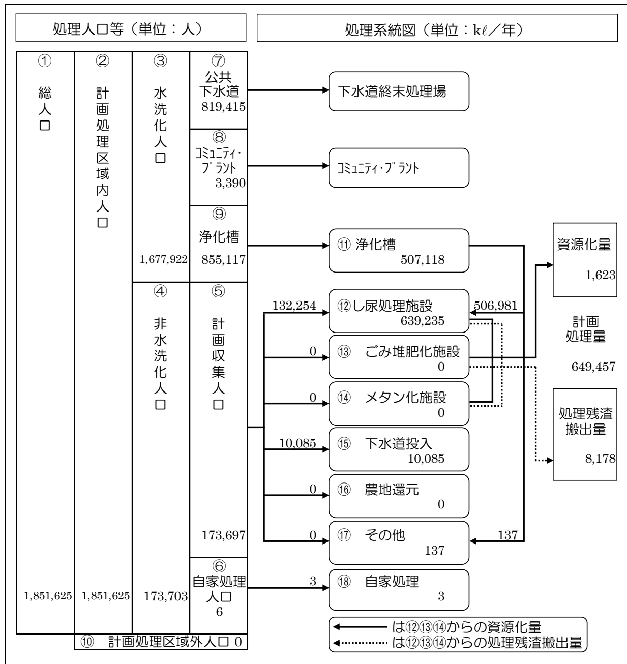
資料7-11 し尿処理のフロー図（平成24年度）
