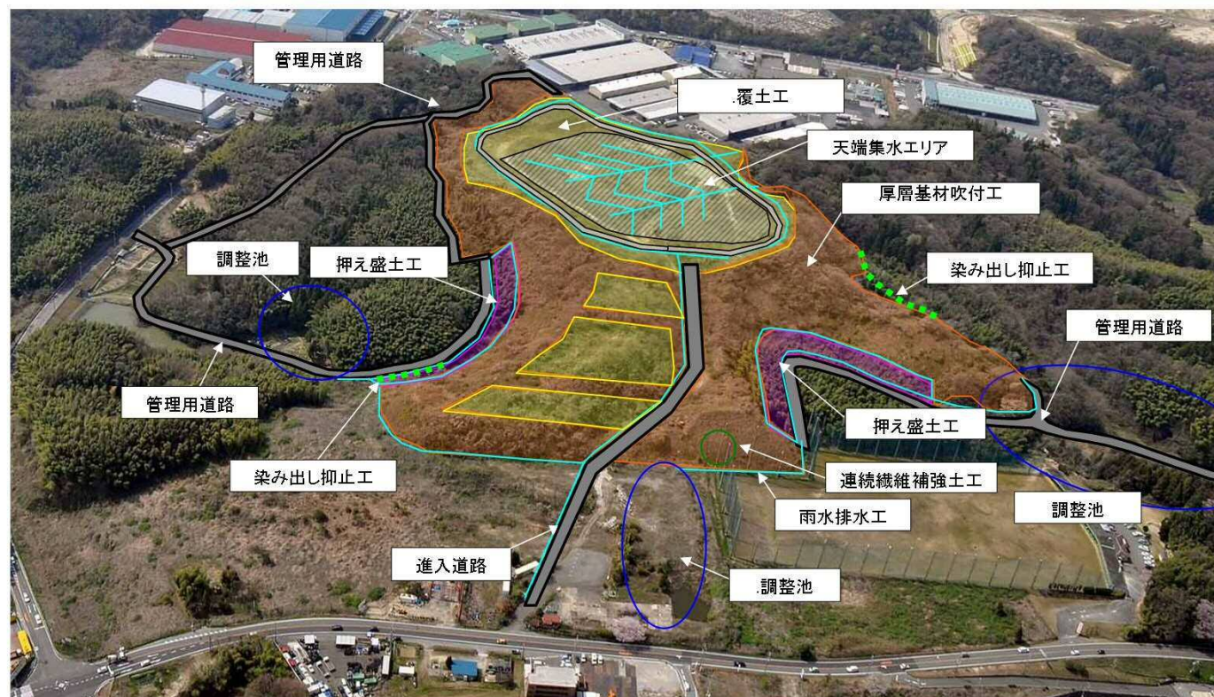
支障除去対策工のイメージ図
