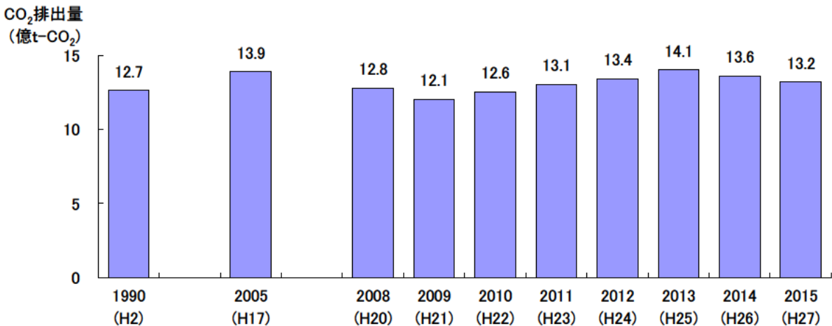
参考 日本における温室効果ガス排出量の状況
