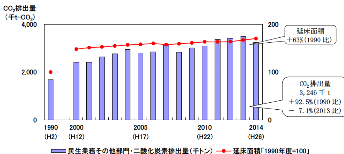
図 5-3-1 二酸化炭素排出量と延床面積の推移
