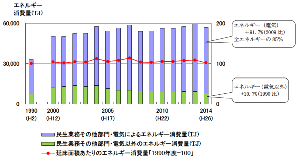
図5-3-3 エネルギー消費量の内訳と延床面積当たりのエネルギー消費量の推移
