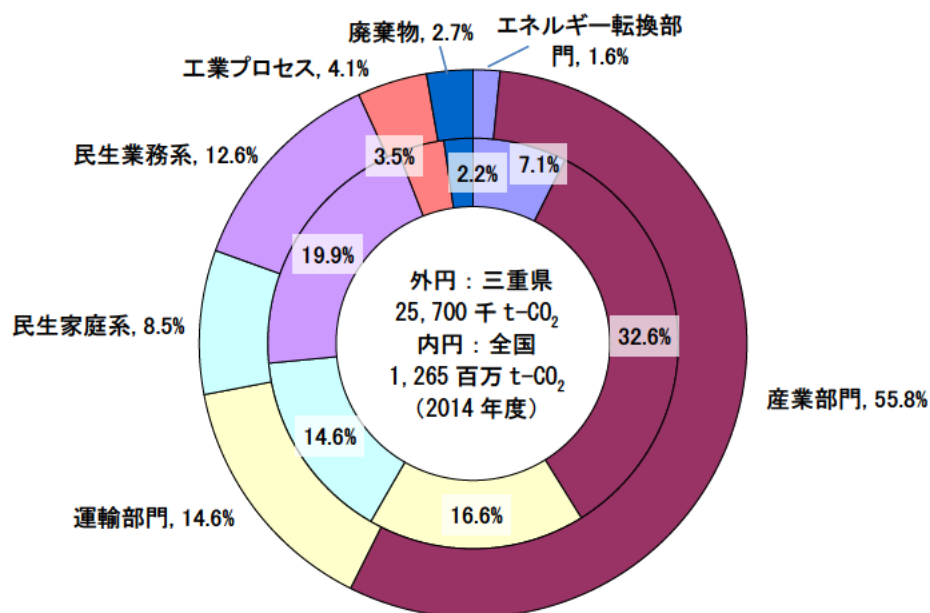
図 4-1-1 部門別二酸化炭素排出量の構成比 (外円：三重県、内円：全国)
