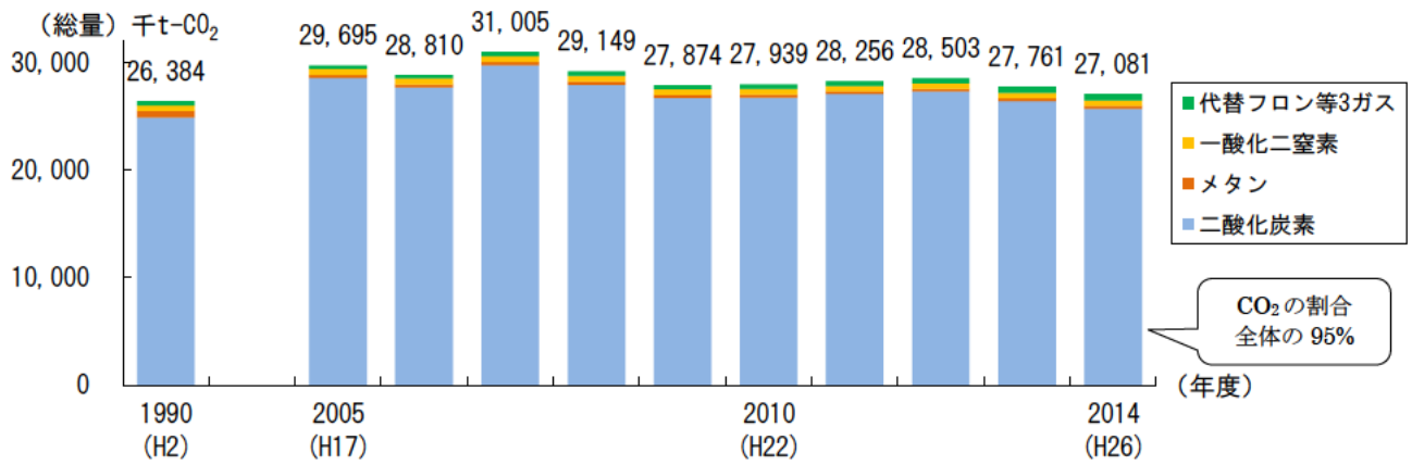
図 2-1 三重県における温室効果ガス排出量の推移
