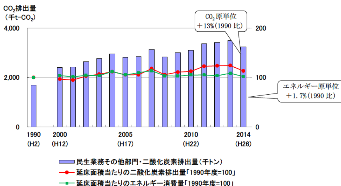
図 5-3-2 延床面積当たりの二酸化炭素排出量・エネルギー消費量の推移
