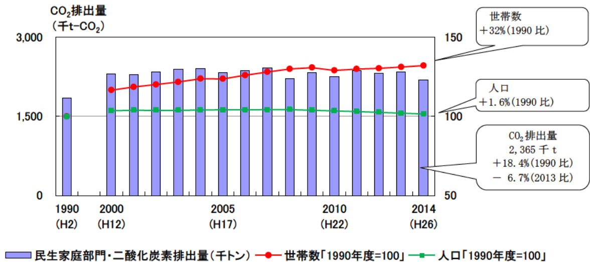
図 5-4-1 二酸化炭素排出量と人口・世帯数の推移
