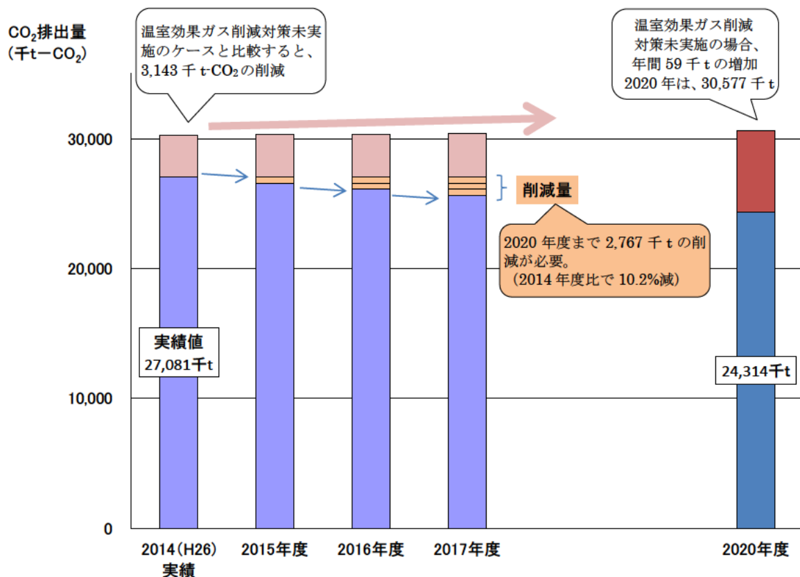
図 3 温室効果ガス排出量の削減状況
