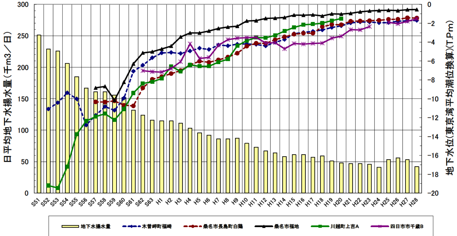
図-2 規制区域内地下水揚水量と主な地点の地下水位の経年変化
