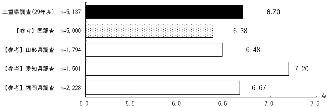
図表 2-1-3 (参考)国及び他県における類似の調査結果(「幸福感」を10点満点で尋ねる調査)
