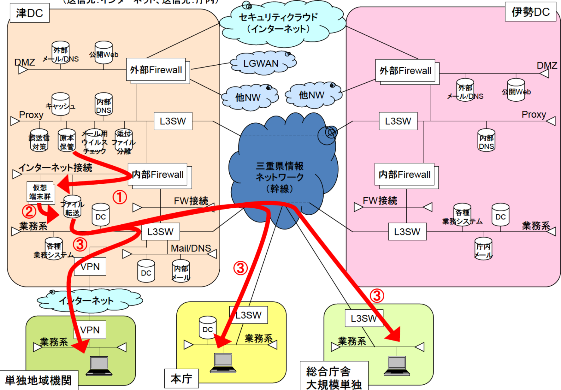
別紙3-2:三重県行政WAN インターネットメールフロー案(原本保管サーバからのファイル抽出及び転送) (送信元:インターネット、送信先:庁内)
