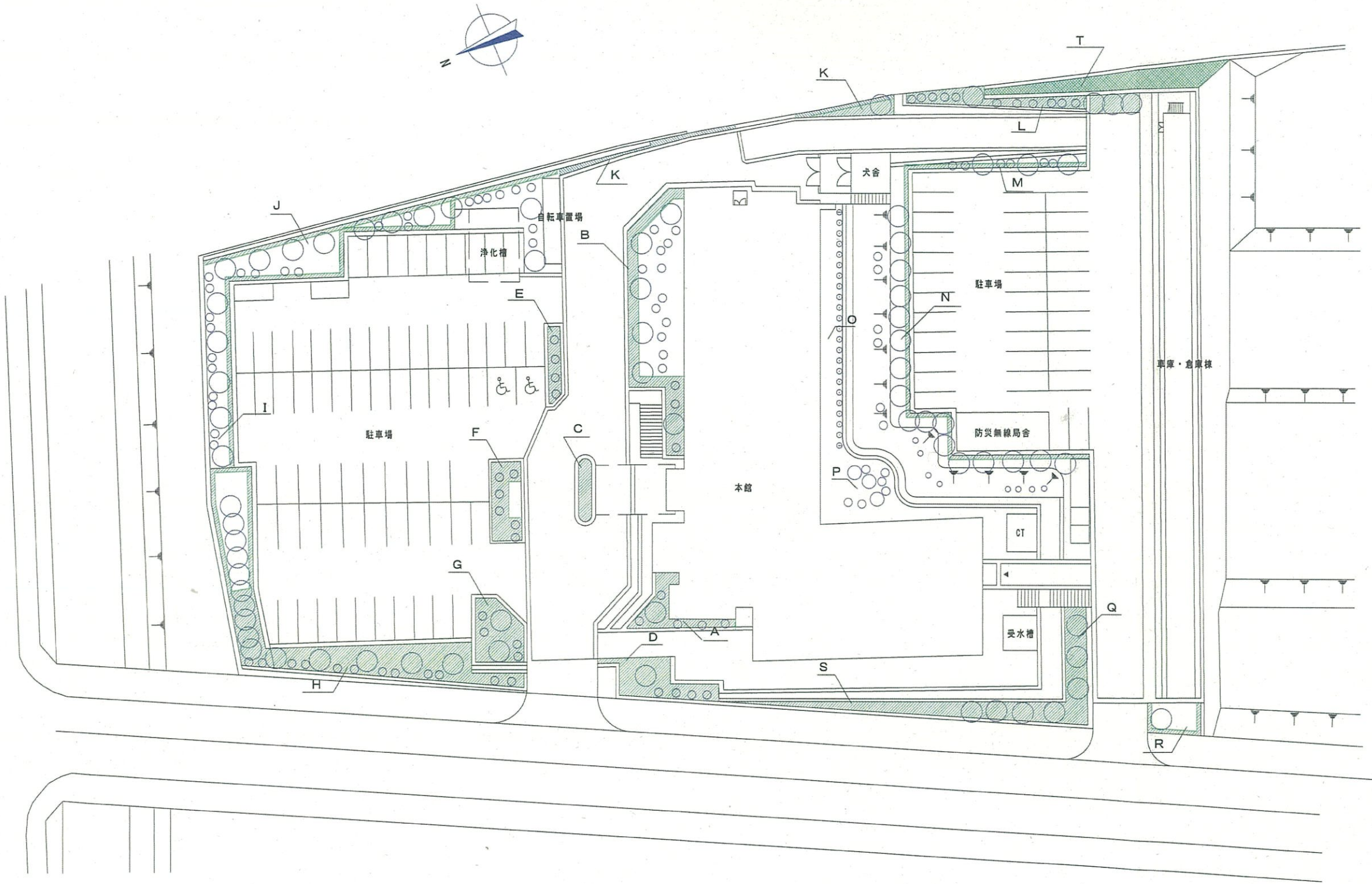
志摩庁舎配置図 1 : 600
