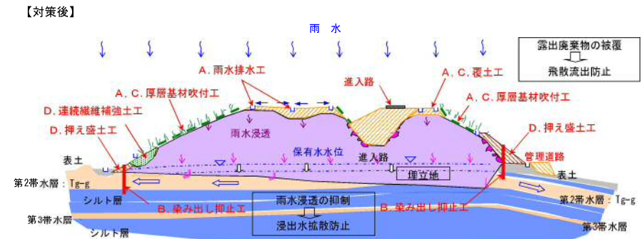
支障除去対策工の概念図
