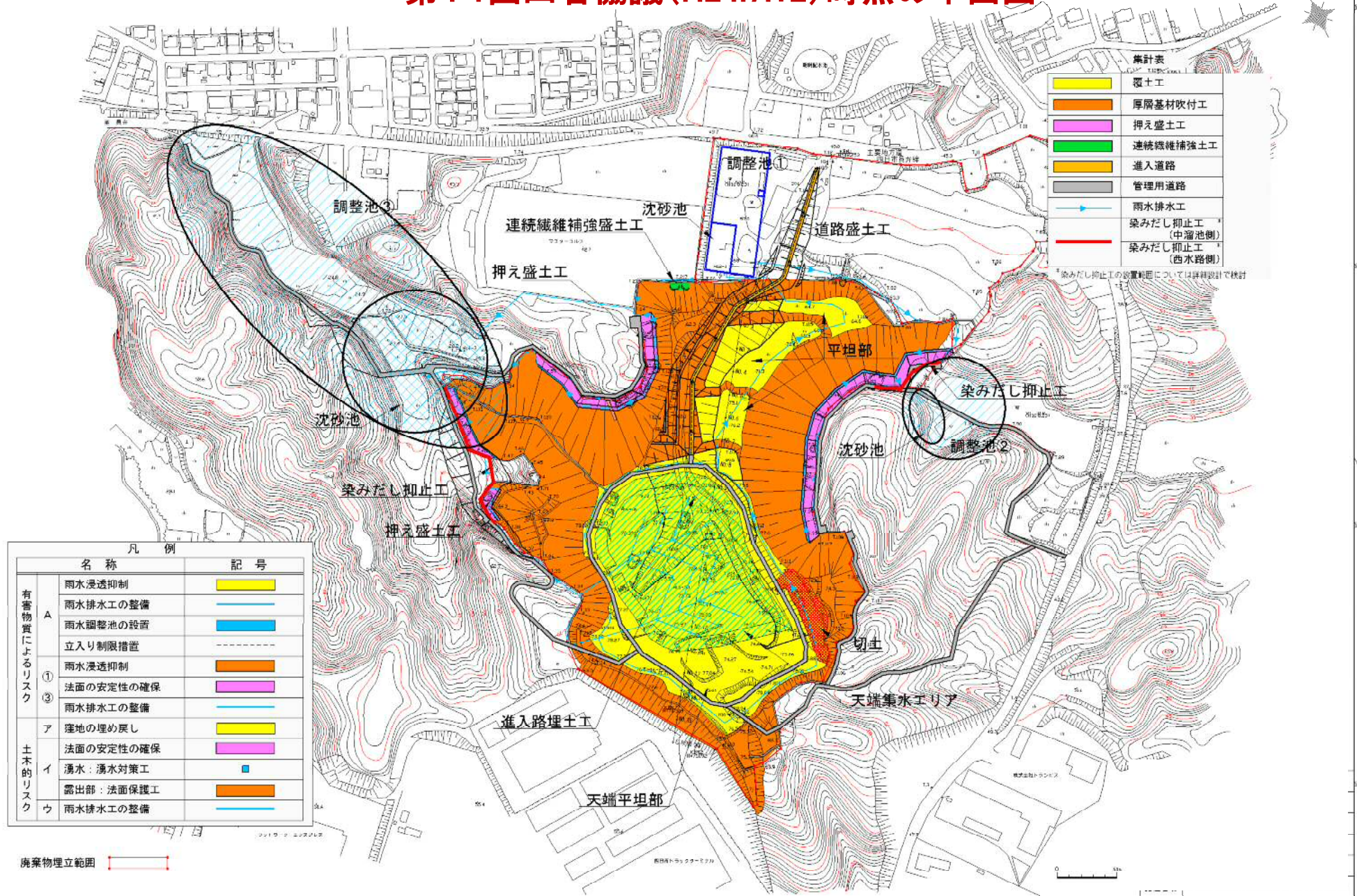
(2) 支障除去対策工全体計画平面図
