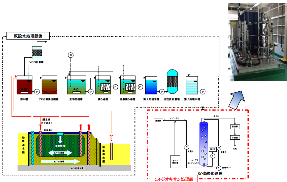
図 4 - 6 水処理施設改良図
