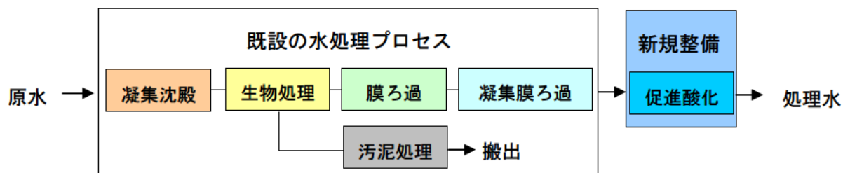
図4-4 1,4-ジオキサン分解のための水処理フローの概略
