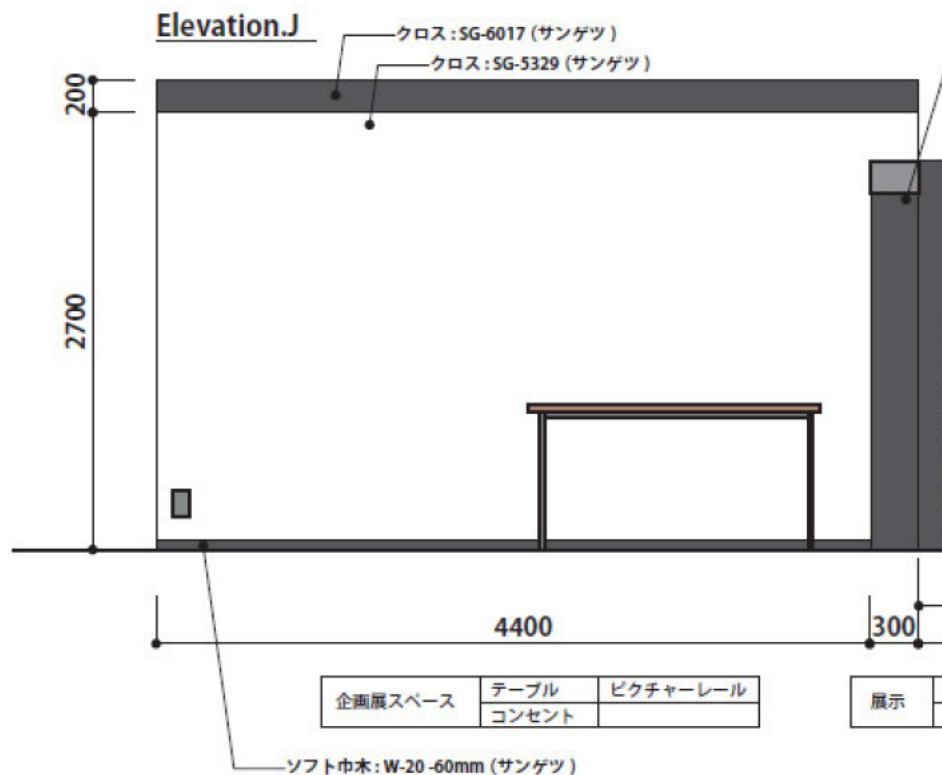
(展示スペース立面図)
