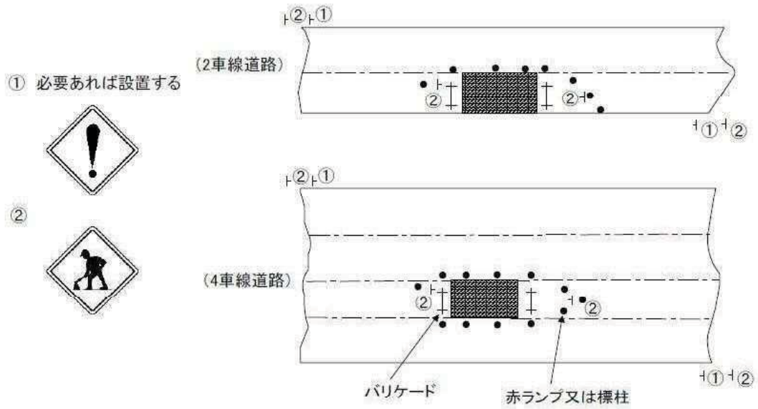
参考（２） 工事中迂回路の標示例（市街部の場合） （進行方向に対する標識の設置例を示す）
