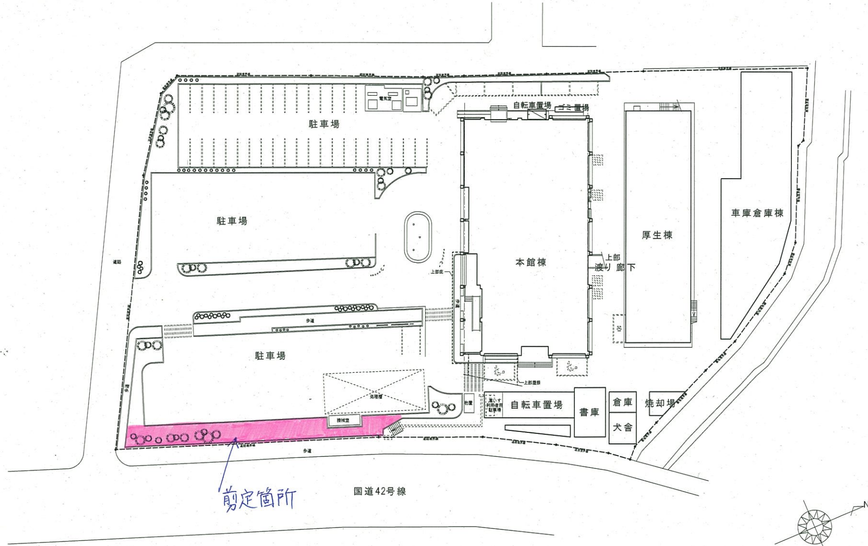
尾鷲庁舎 配置図 S:1/500
