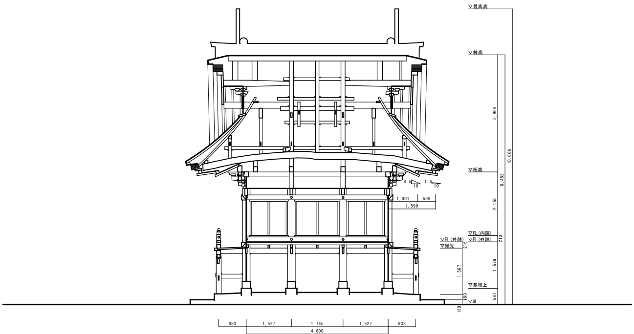
桁行断面図 (C断面)
