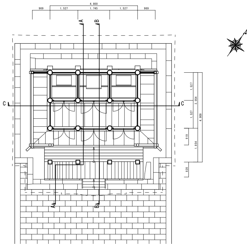
平面図
