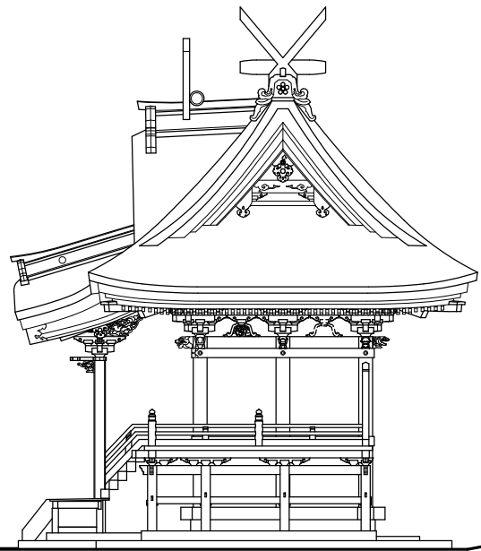
立面図（東面）
