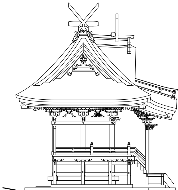
立面図（西面）
