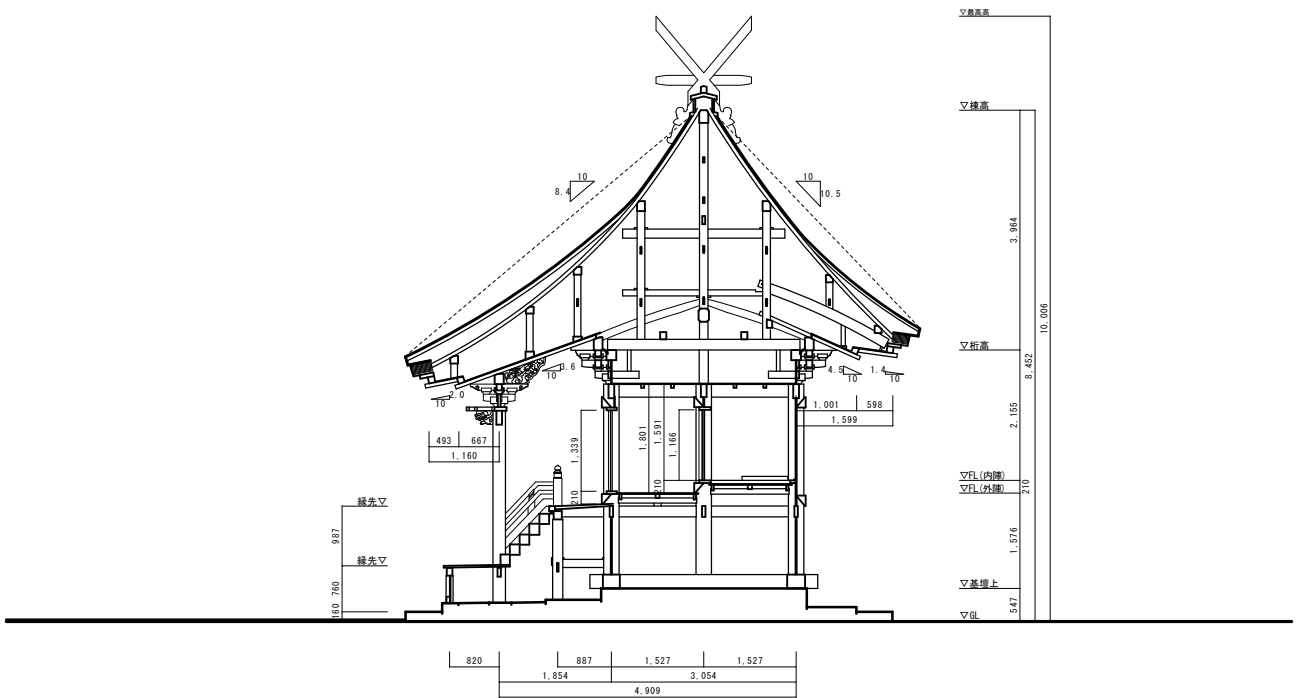
梁間断面図 (A断面)
