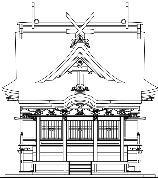
立面図（南面）
