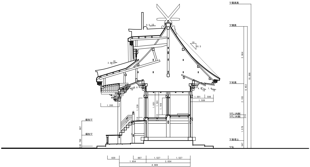
梁間断面図 (B断面)
