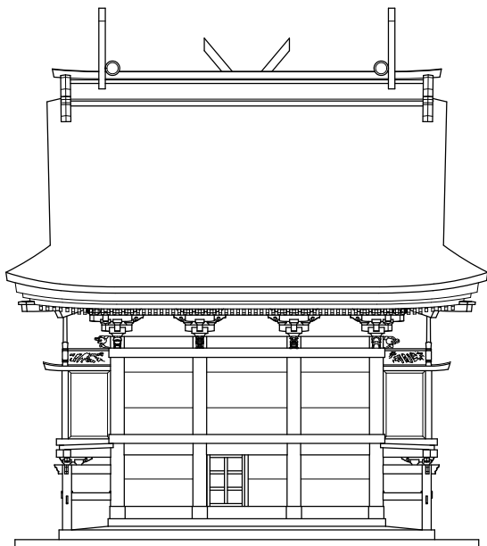
立面図（北面）
