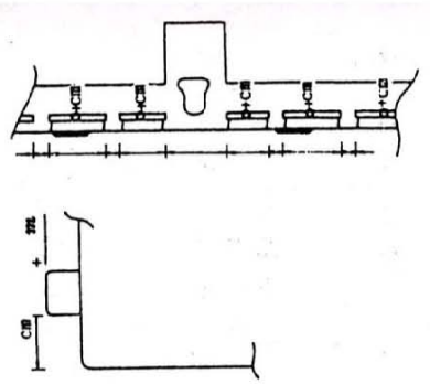
車止測定位置図
