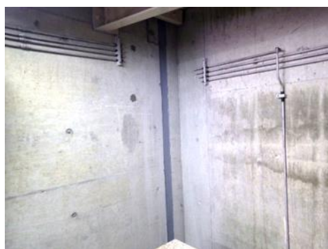
↑ 耐震スリット
