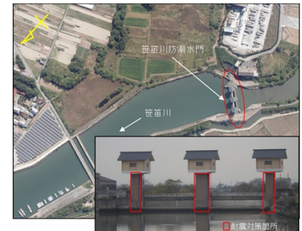
笹笛川防潮水門耐震対策 (三重県)
