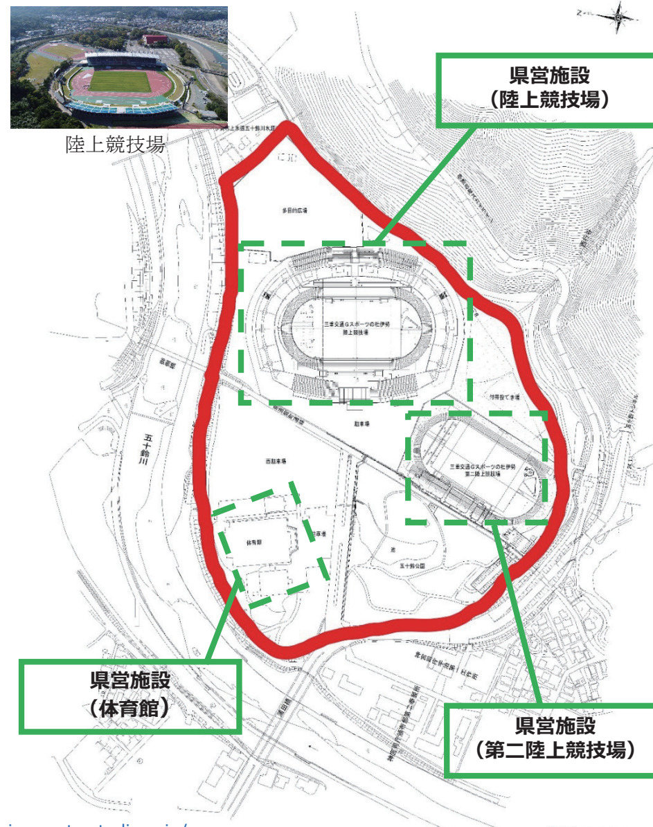
都市公園（五十鈴公園） 平面図 （赤線が都市公園の境界）
