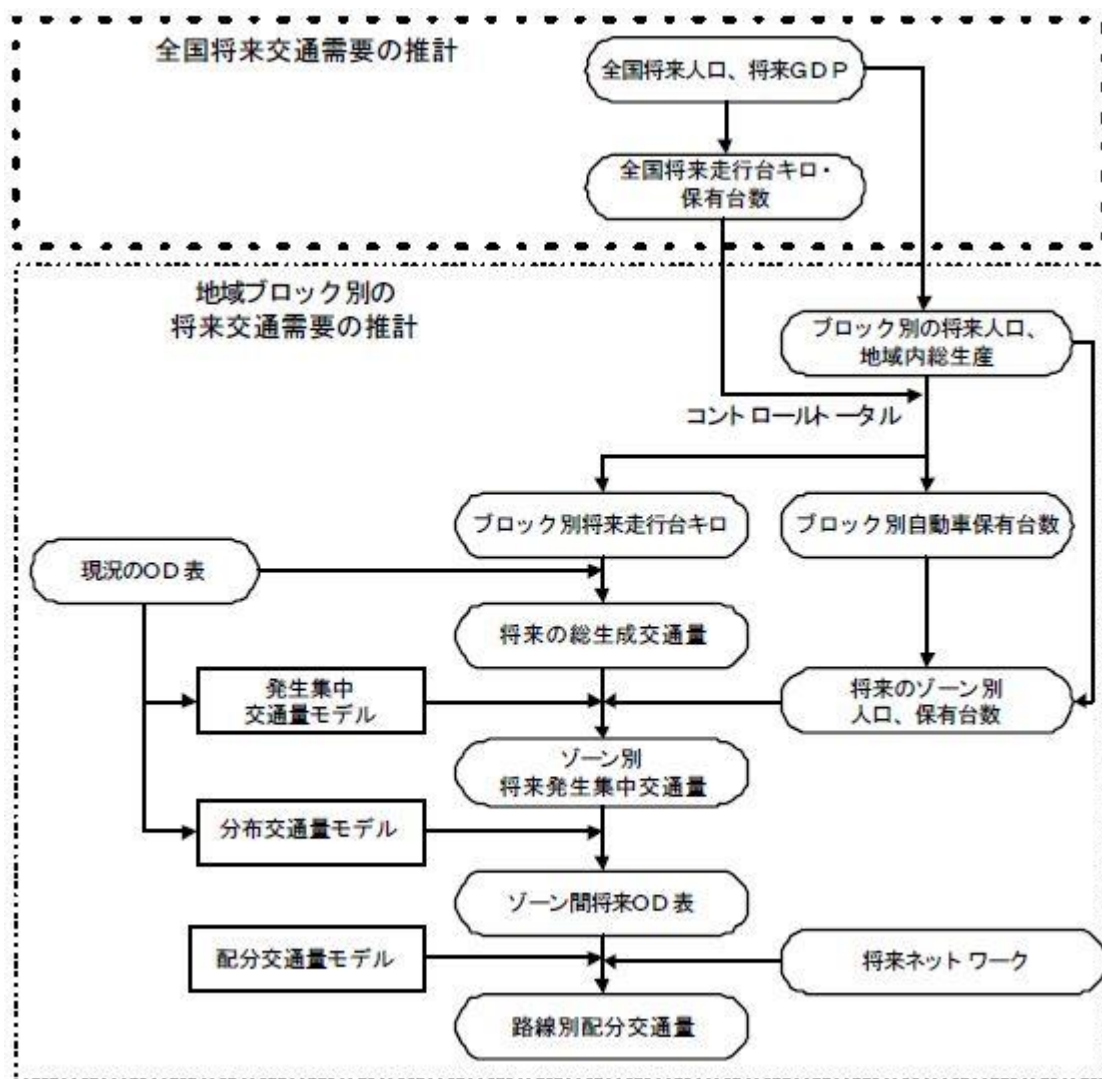
図 1 道路計画における将来交通需要推計の手順
