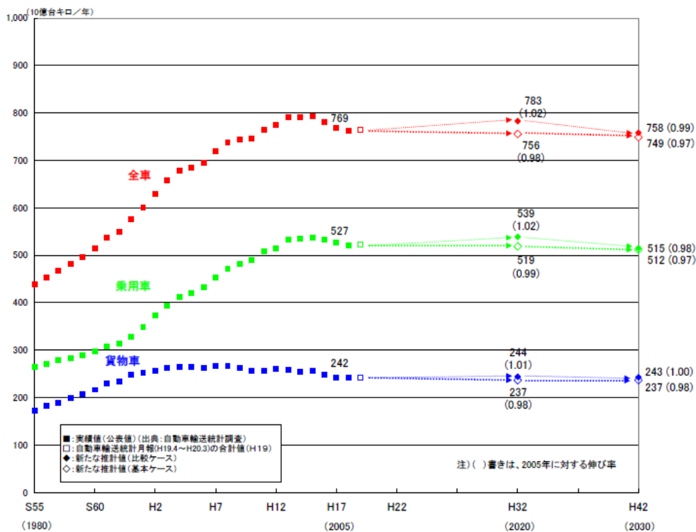
図2 全国交通量 (走行台キロ) の実績値と推計値
