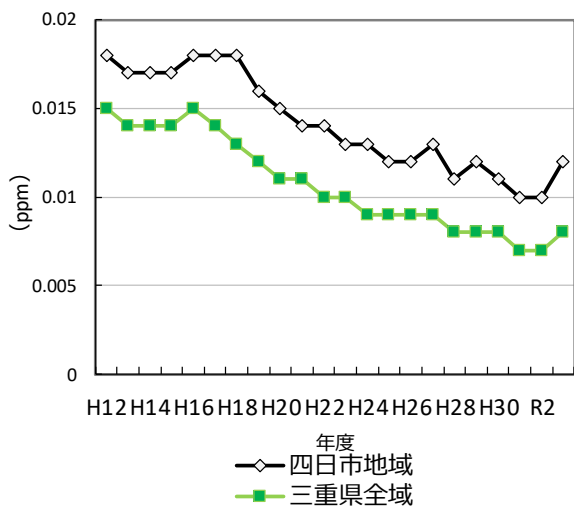
図 2-4-2 二酸化窒素の経年変化（一般局の年平均値）
