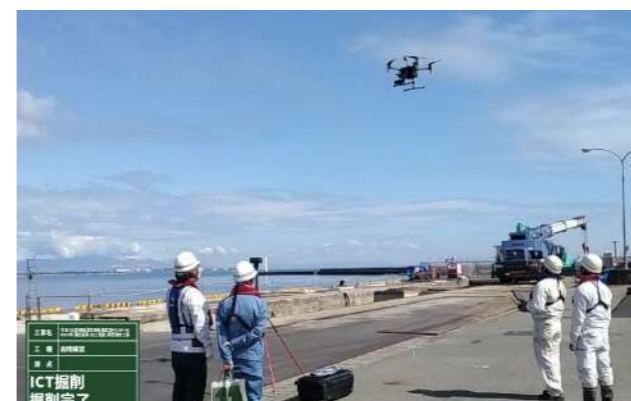
ドローンによる起工測量
