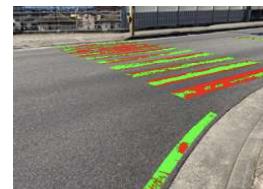
AI路面標示劣化検知システム
