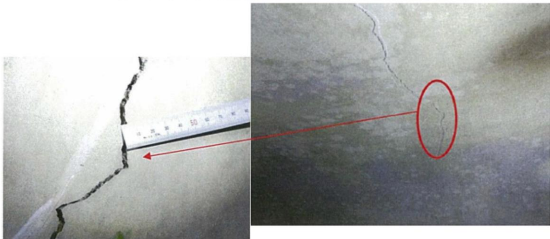
付写真-2.3.1 覆エスパンの中間付近に発生したひび割れの例
