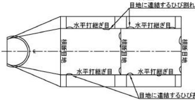
矢板工法（覆工打込み方法：逆巻き）の例
