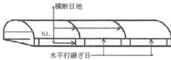
矢板工法（覆工打込み方法：逆巻き）の例
