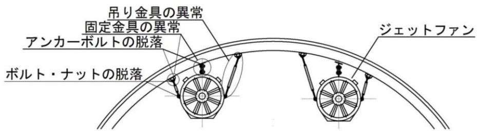
付図-2.5.1 附属物の異常発生箇所
