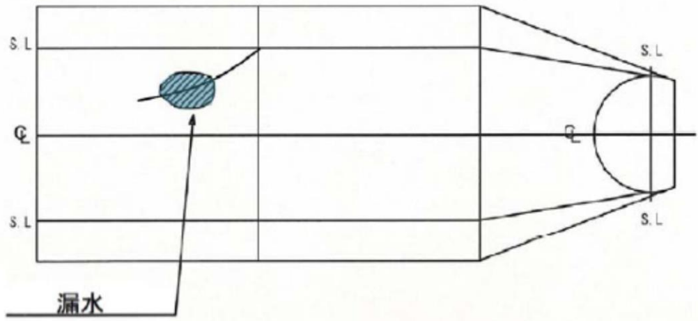
付図-2.4.4 ひび割れからの漏水位置の例
