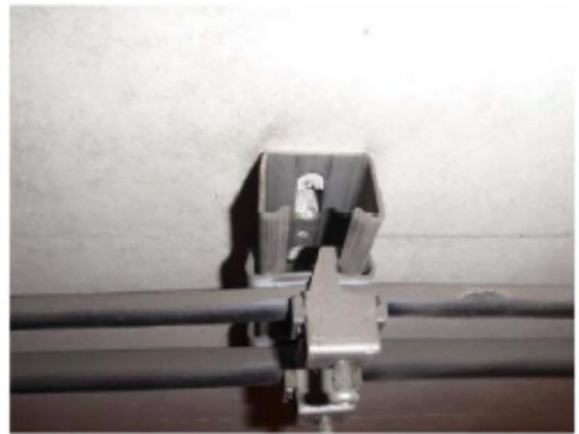
付写真-2.5.1 固定金具の腐食とアンカーボルトの脱落の例
