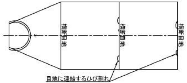
山岳トンネル工法（覆工打込み方法：全断面）の例
