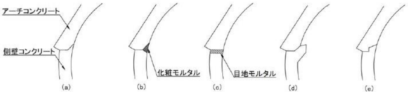
付図-2.1.3 逆巻き工法の水平打ち継ぎ目の種類
