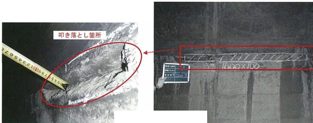
付写真-2.1.2 逆巻き工法の水平打継ぎ目と化粧モルタル、目地モルタルの施工状況
