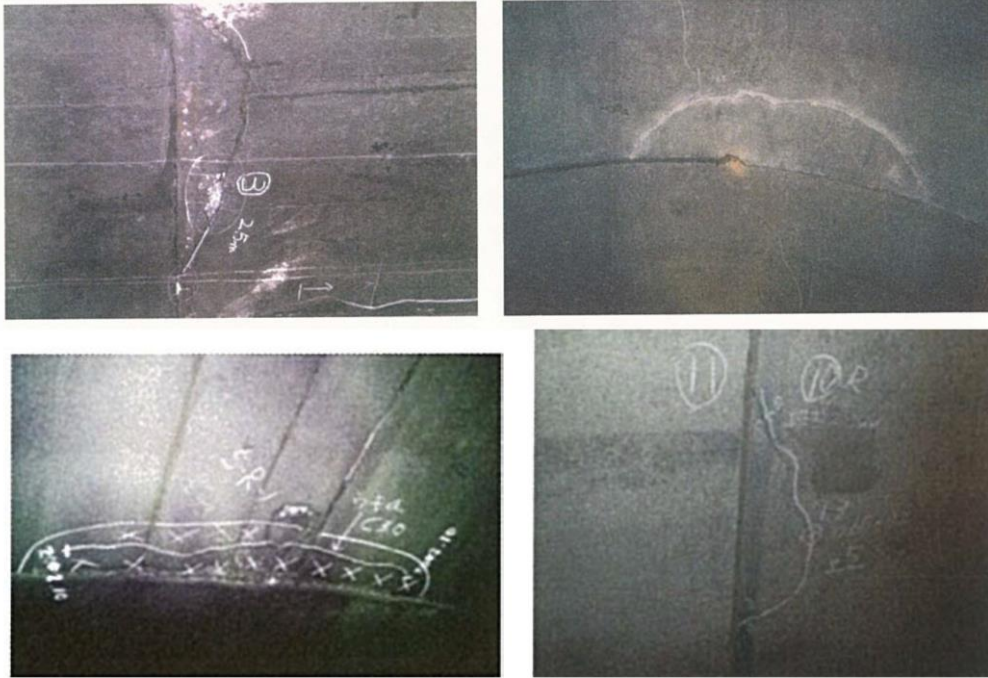
付写真-2.1.1 横目地の天端付近に発生した半月状のひび割れの例
