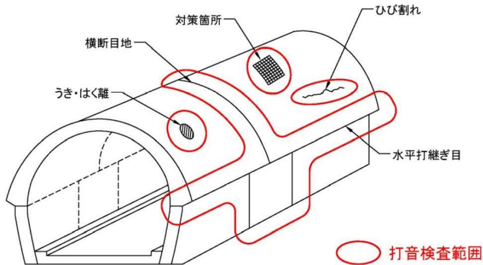
図 重点的に確認する範囲のイメージ
