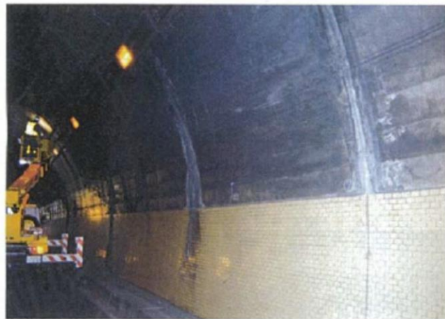
付図-2.3.1 覆エスパンの中間付近に発生する変状の例
