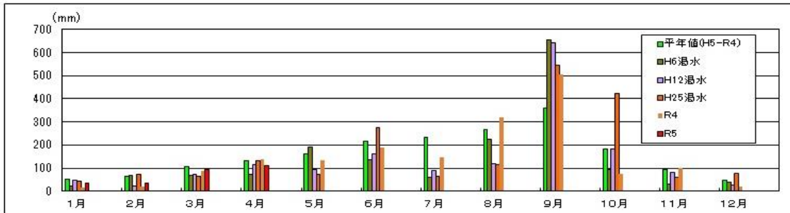
令和5年 八手俣川上流（上多気地点）降雨状況 [速報値]
