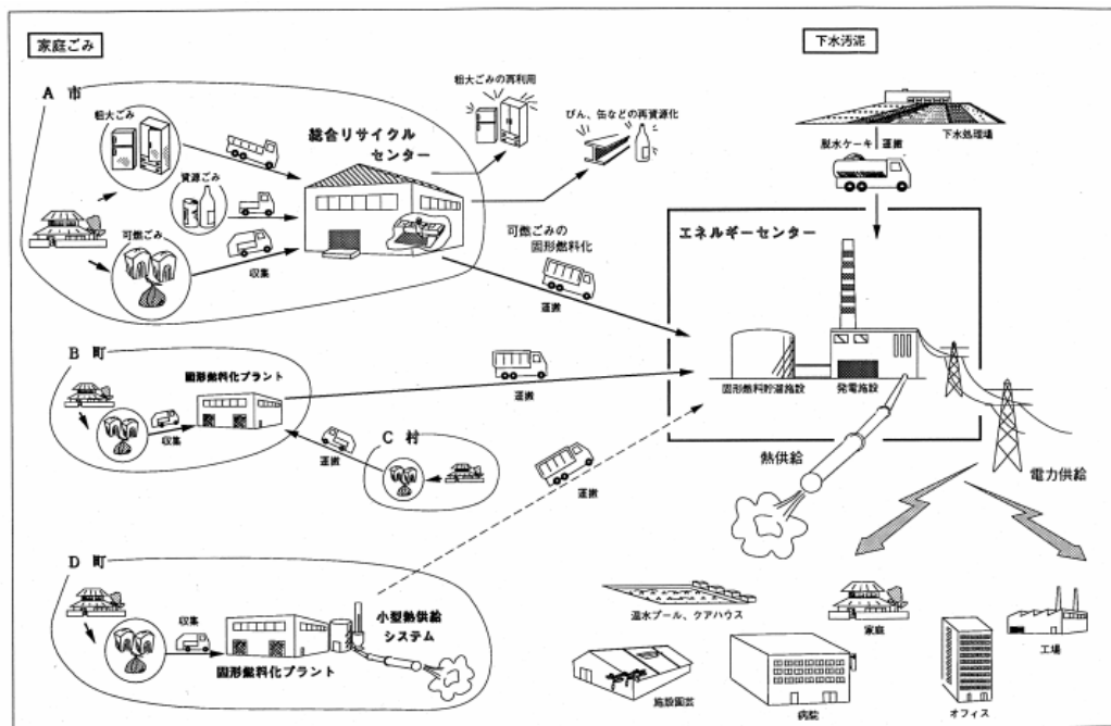
RDF発電構想イメージ図
