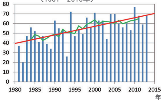
図-1-14 桑名における真夏日の年間日数の変化 (1981～2013年)
