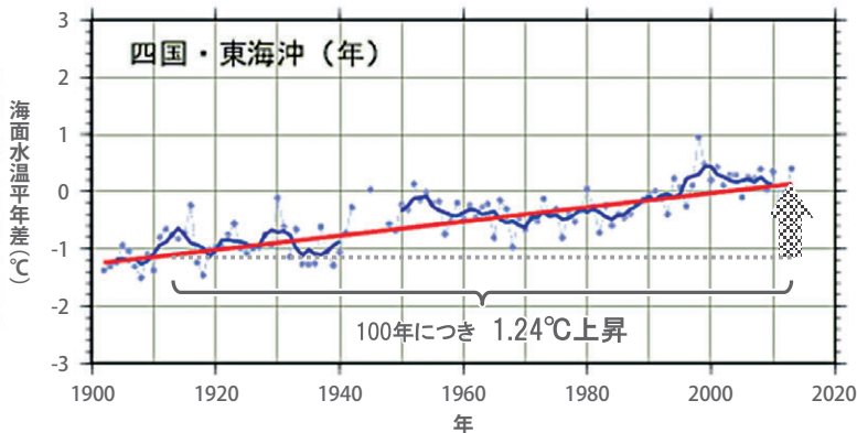
図-1-18 四国・東海沖の海域平均海面水温年差(1902~2013年)
