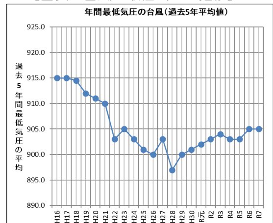
【図表 台風の最低気圧の推移】
