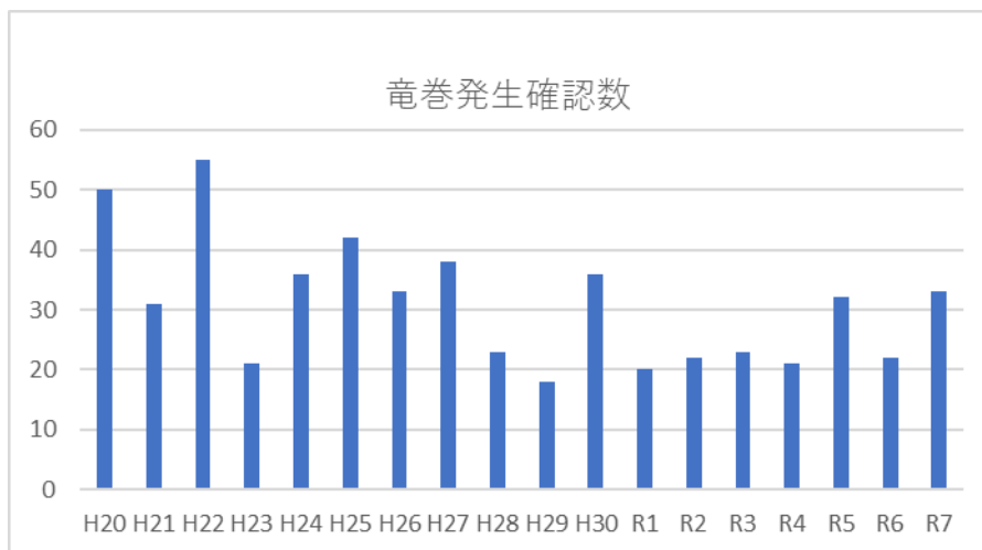
【図表 全国の竜巻発生確認数】
