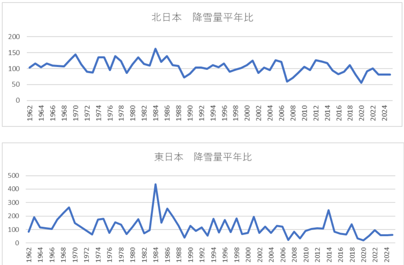
【図表 降雪量の平年比の推移】
