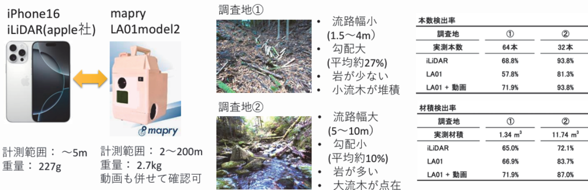
図-6. 地上3次元計測技術による流木量調査の比較検証
